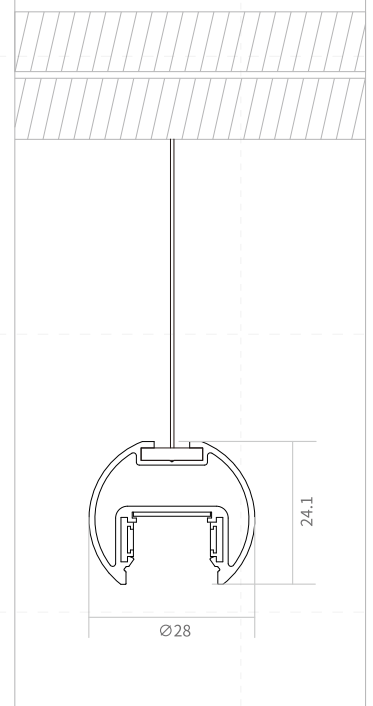
TLS-MSR15X0 Pendant Track
