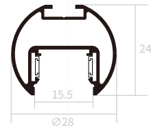
TLS-MSR15X0 Pendant Track
